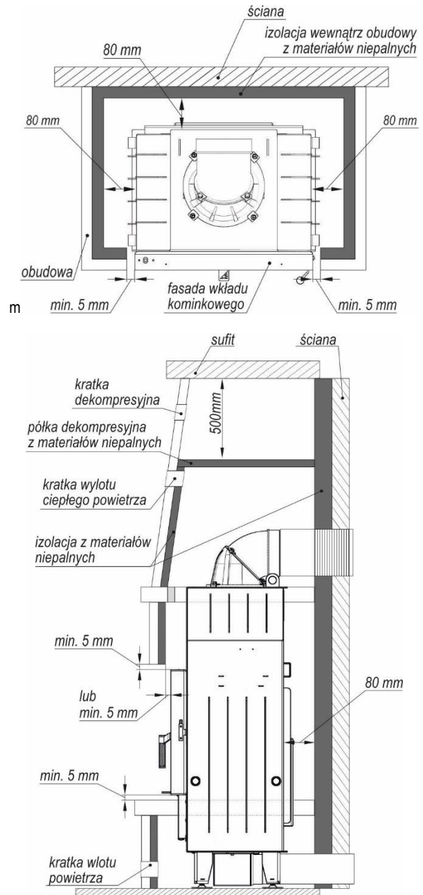
Rysunek 3. Przykładowa zabudowa wkładu kominkowego.
