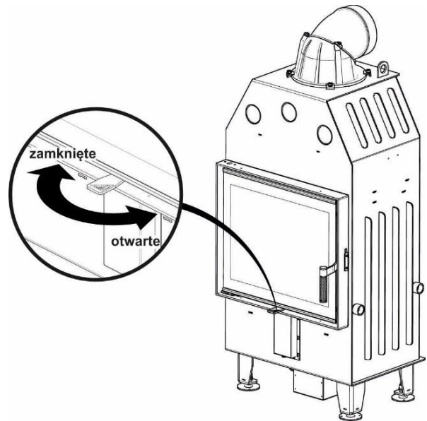
Rysunek 7. Ustawienie suwaka regulacji dopływu powietrza.
