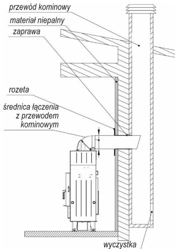
Rysunek 6. Podłączenie wkładu kominkowego do przewodu kominowego.
