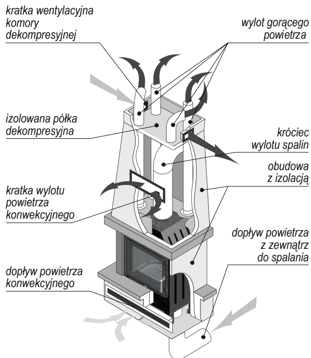
Rysunek 4. System dystrybucji gorącego powietrza.
