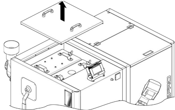
KROK 1. Podnieść pokrywę maskującą wyczystki górnej
