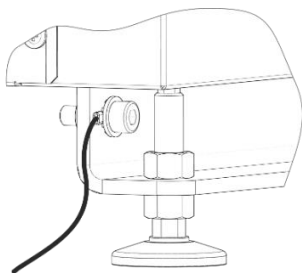
Rysunek 13. Uziemiaenie kotła.
