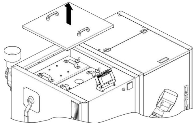
KROK 1. Podnieść pokrywę maskującą wyczystki górnej
