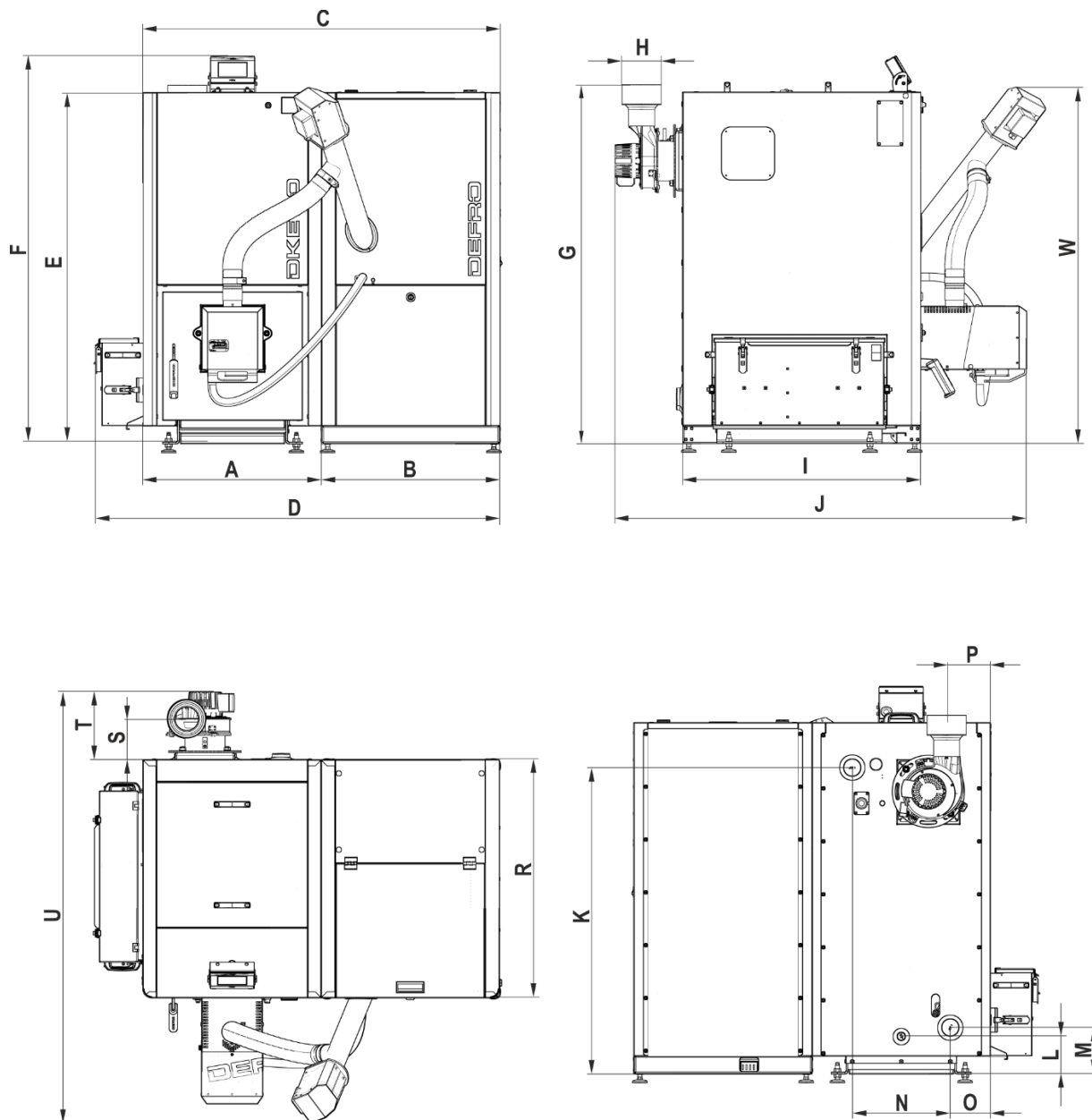
Rysunek 2. Podstawowe wymiary kotła KOMPACT EKOPELL F.
