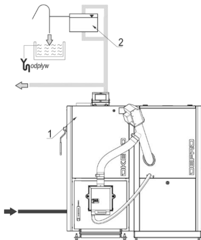
Rysunek 8. Przykładowy schemat zabezpieczeń kotła KOMPACT EKOPELL / KOMPACT EKOPELL F: 1-kocioł; 2-otwarte naczynie zbiorcze.
